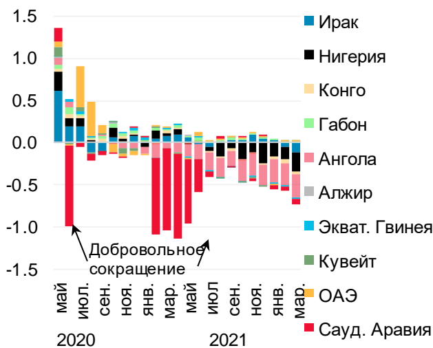
Рисунок 18. Отклонение добычи нефти ОПЕК от квот («+» – превышение квот), млн б/с
