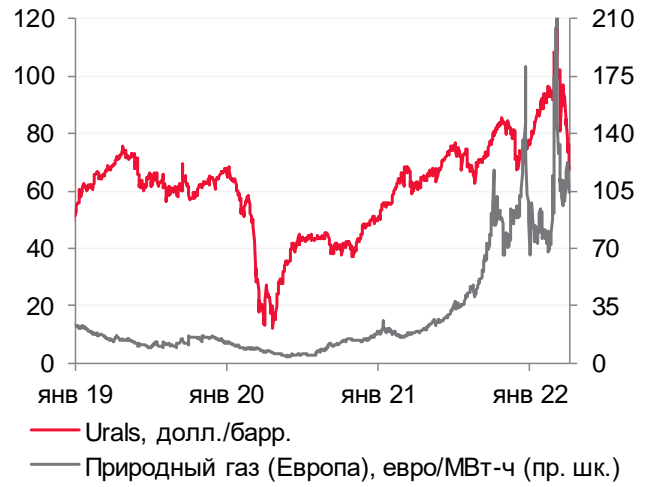
Рисунок 17. Цена нефти Urals и природного газа в Европе
